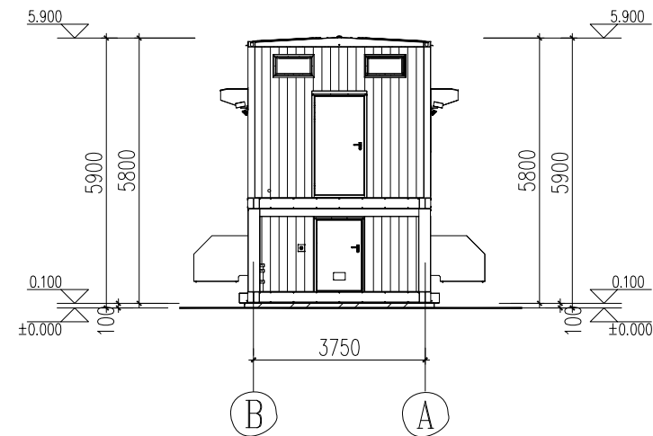
换电站左立面 1:100
